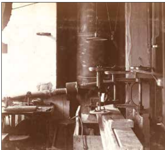
Машины для распиливания (слева) и шлифовки и полировки камней
